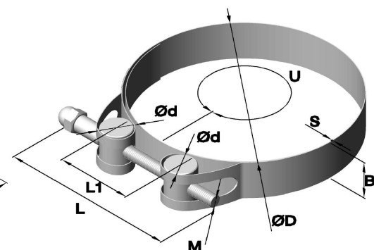
Serie 1701 Gelenkbolzenband
