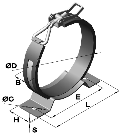
Serie 1501 Rohrspannverschluss mit Konsole und C-Gummiprofil
