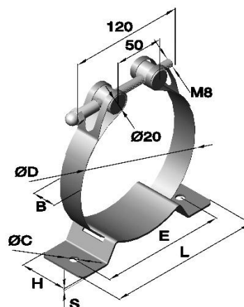
Serie 1901 Typ1 Rohrspannverschluss mit Konsole und Gelenkbolzen
