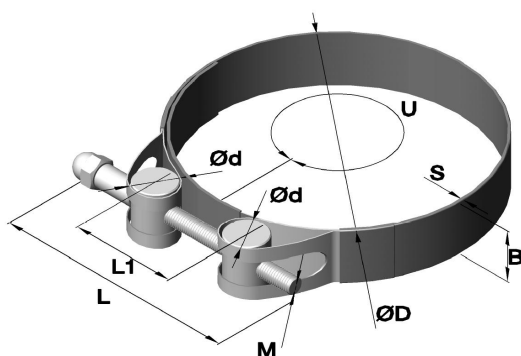
Serie 1801 Gelenkbolzenband mit Kunststoffummantelung
