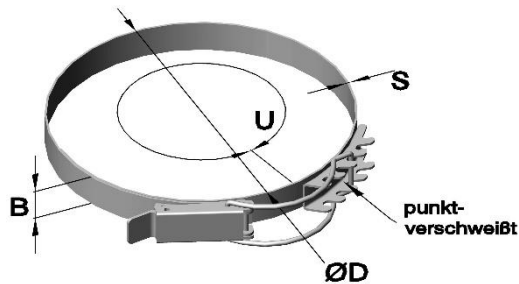
Serie 1201 Spannband mit und ohne Feder
