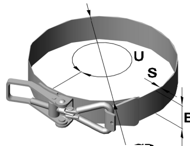
Serie 1301 Spannband
