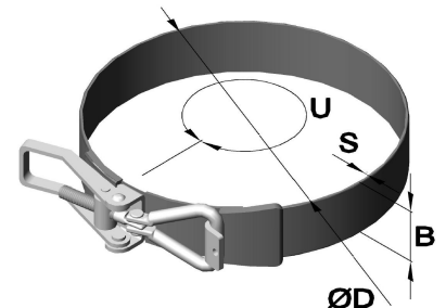
Serie 1401 Spannband mit Kunststoffummantelung
