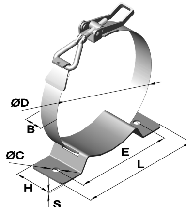
Serie 1601 Rohrspannverschluss mit Konsole
