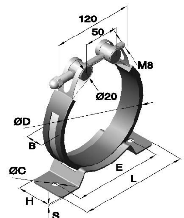
Serie 1901 Typ2 Rohrspannverschluss mit Konsole, C-Gummiprofil und Gelenkbolzen
